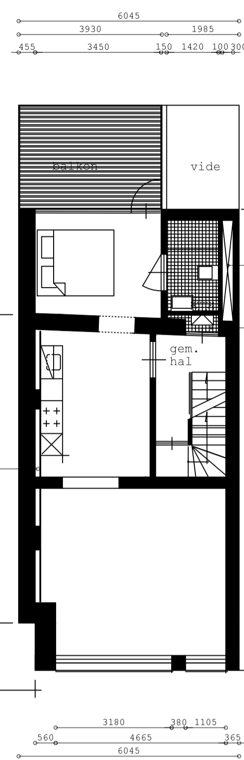
eerste verdieping appartement II (schaal 1:100)
