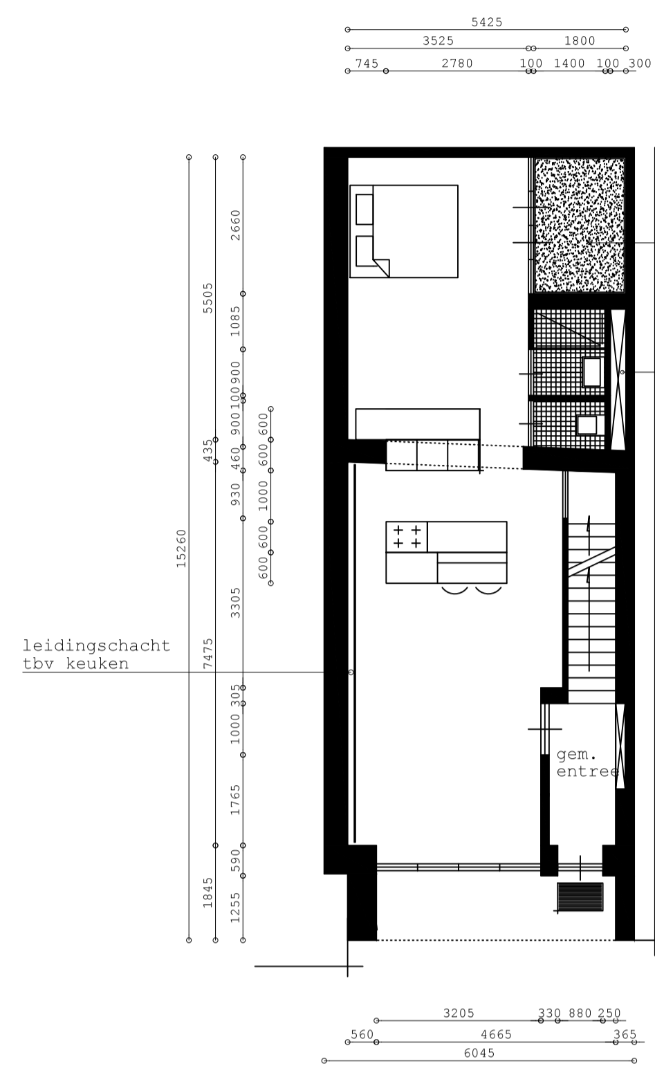
begane grond appartement I (schaal 1:100)
