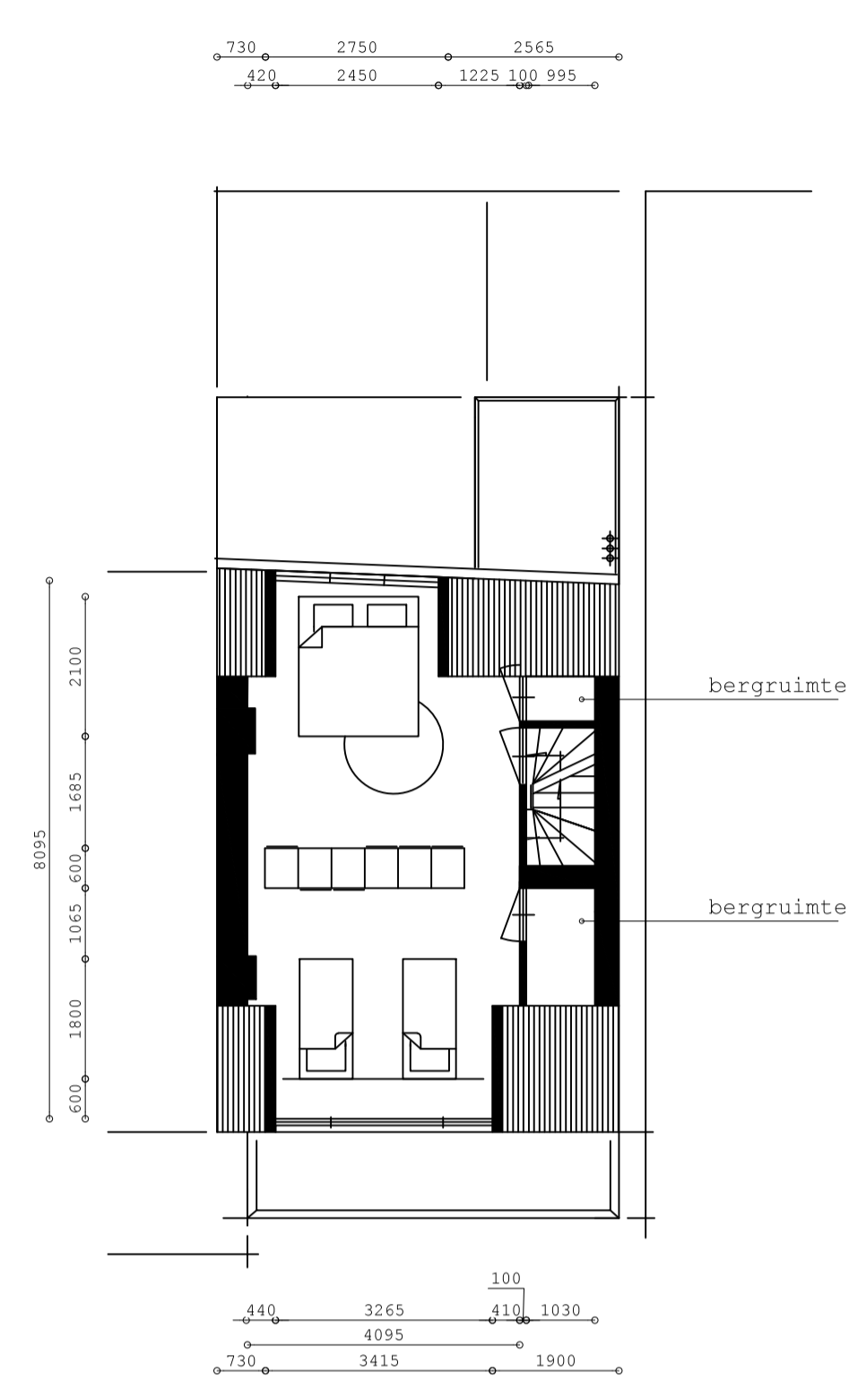
derde verdieping appartement III (schaal 1:100)
