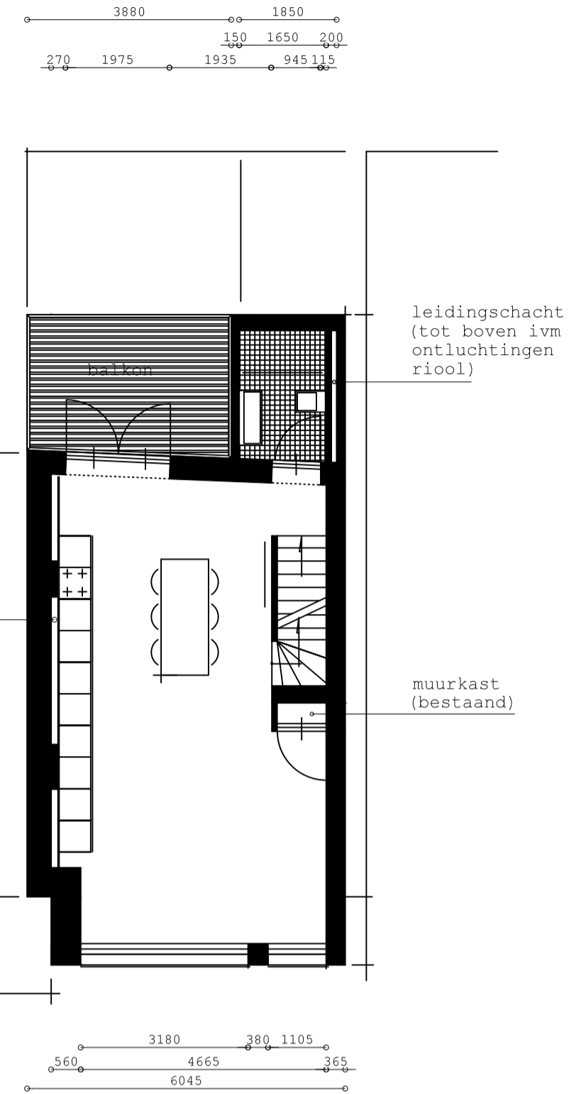
twede verdieping appartement III (schaal 1:100)
